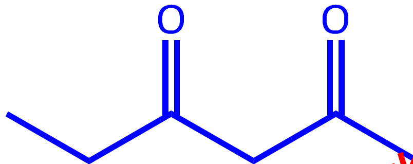
Hexane-2,4-dione
