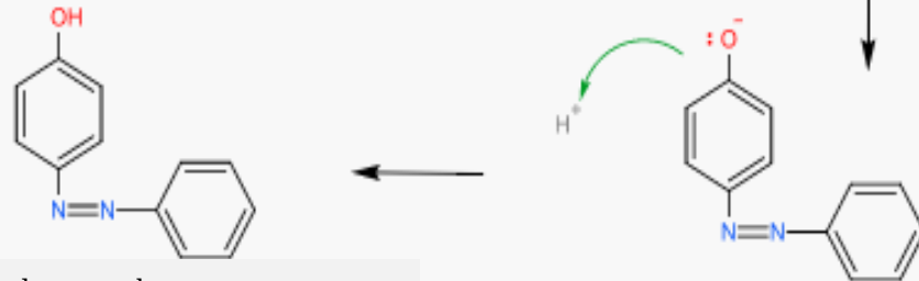
P- hydroxy azobenzene
